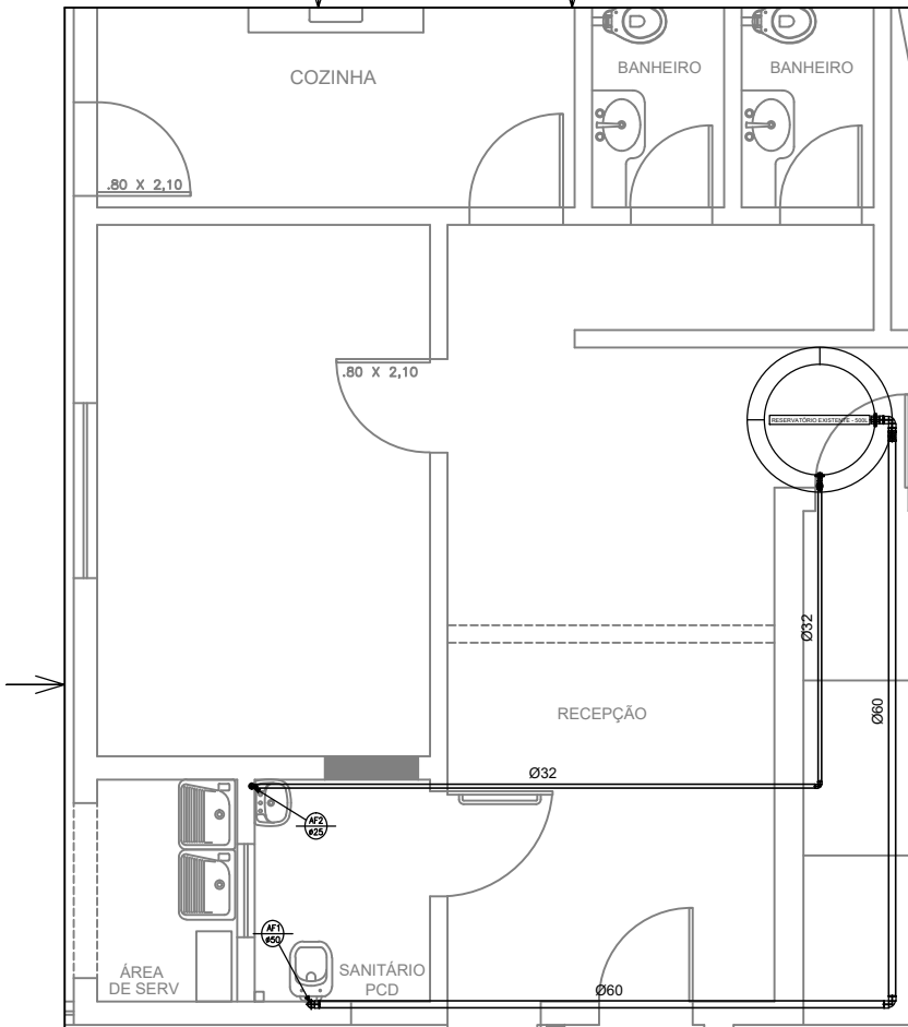
PLANTA ESCALA: 1/50
